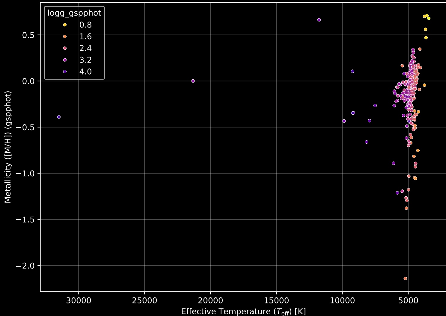
APOGEE DR17 Field: [355-08] Stellar Population Parameters (n= 288)
